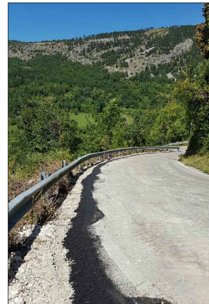
F.4: Ripristino scavo con binder
